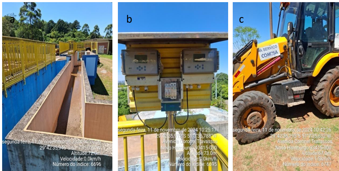
Figura 2: Obras de expansão da ETA de Novo Hamburgo. a) Vista da nova entrada de água bruta para tratamento; b) novos equipamentos de medição instalados; c) retroescavadeira a serviço da Comusa.
